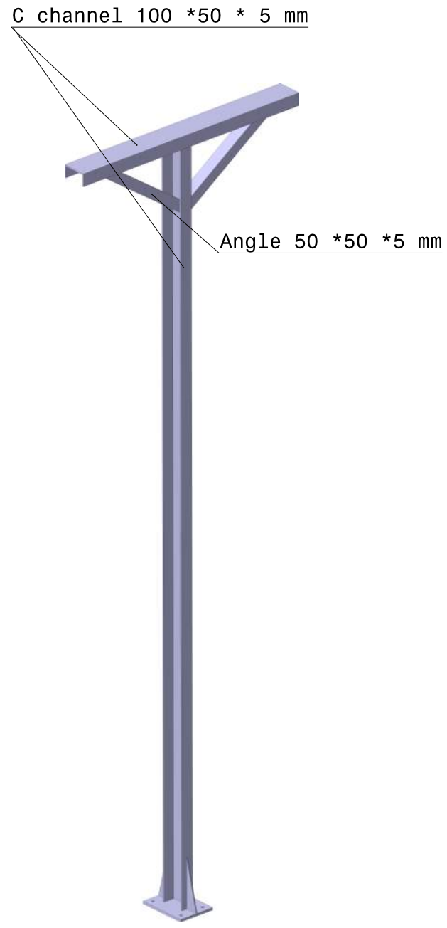
Isometric view Scale: 1:1
