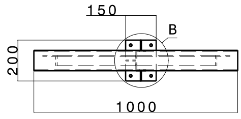
Top view Scale: 1:1
